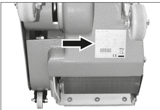
Abb. 2 Typenschild unten am Maschinengehäuse.
