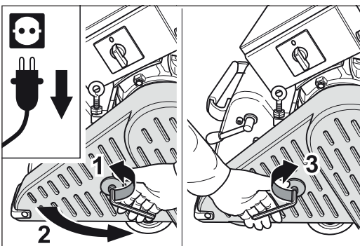
Abb. 3 Zum Ablesen des Maschinentypenschildes bei Maschinen bis August 2022: Den Netzstecker aus der Steckdose ziehen und den Riemenschutz öffnen (1 + 2). Nach dem Ablesen den Riemenschutz wieder schließen (3).
