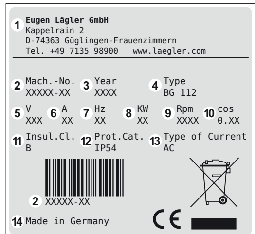
Abb. 6 Angaben auf dem Motor-Typenschild (siehe Haupttext).
