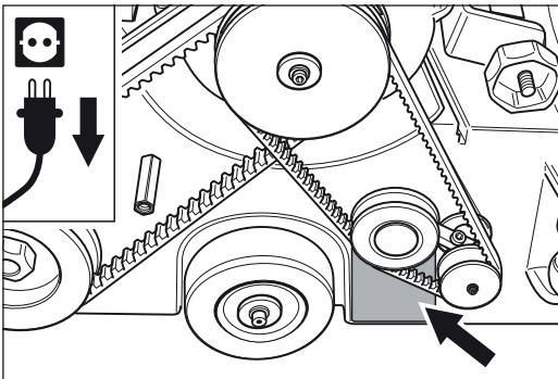
Abb. 2 Maschinentypenschild am Maschinengehäuse unterhalb des Keilriemenspanners (bis August 2022).
