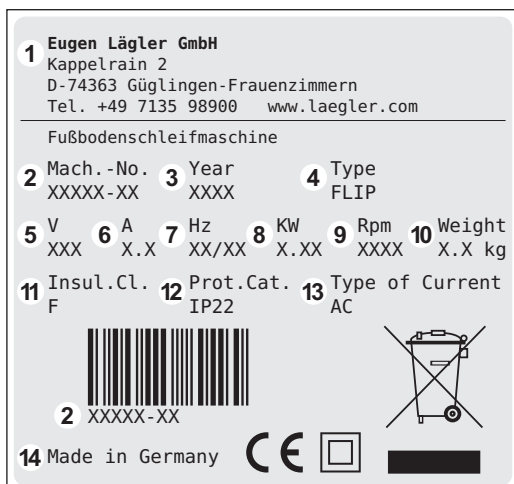
Abb. 2 Angaben auf dem Typenschild (siehe Haupttext).
